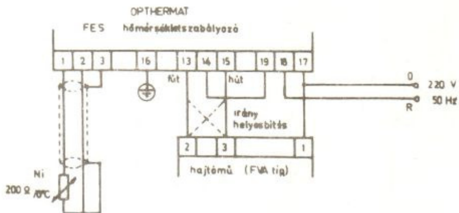
3. ábra FES precíziós szabályozó bekötése
